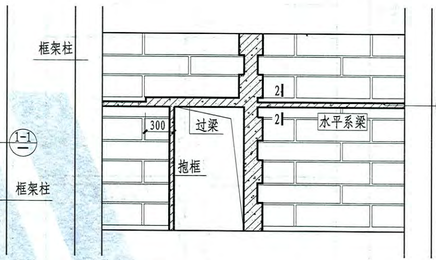
有洞口墙体构造柱设置示意（二）
