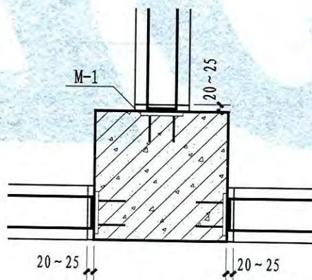
④ 平齐内柱墙
