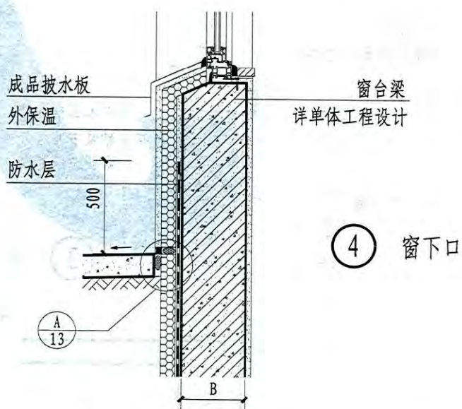
窗上口、窗下口构造详图（三）
