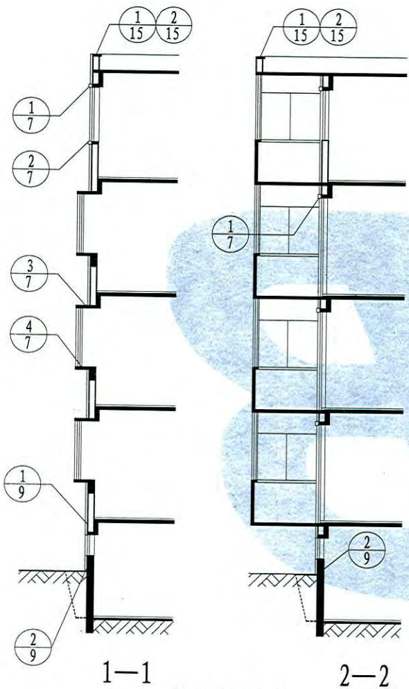
剖面详图索引 (外包墙)
