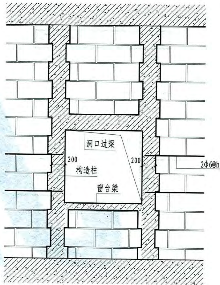
洞口宽度 > 2100 窗洞口做法 (二)
