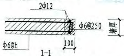
洞口宽度 \leq 2100 窗洞口做法 (一)
