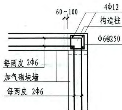
① 构造柱及与墙体拉结图
