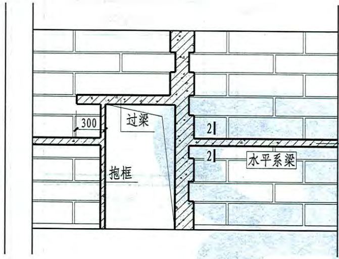
有洞口墙体构造柱设置示意（一）
