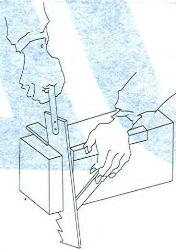
锯块示意
