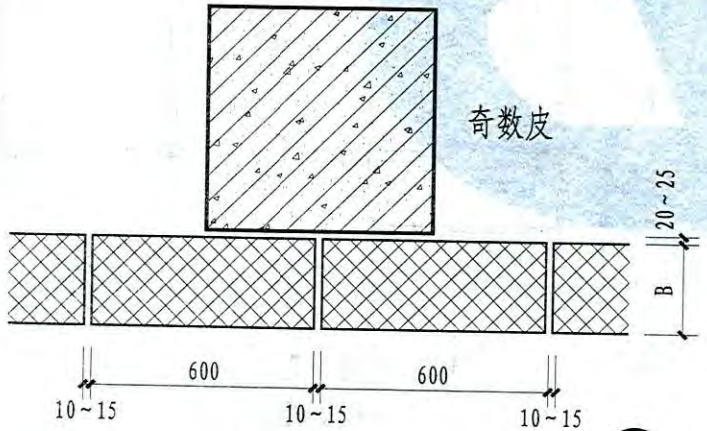
② 边柱处(外包墙)
