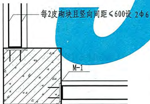
③ 平齐角柱墙
