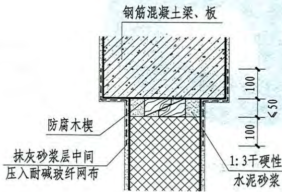
1-1 梁板下墙顶部做法
