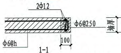
洞口宽度 < 2100 门洞口做法 (一)
