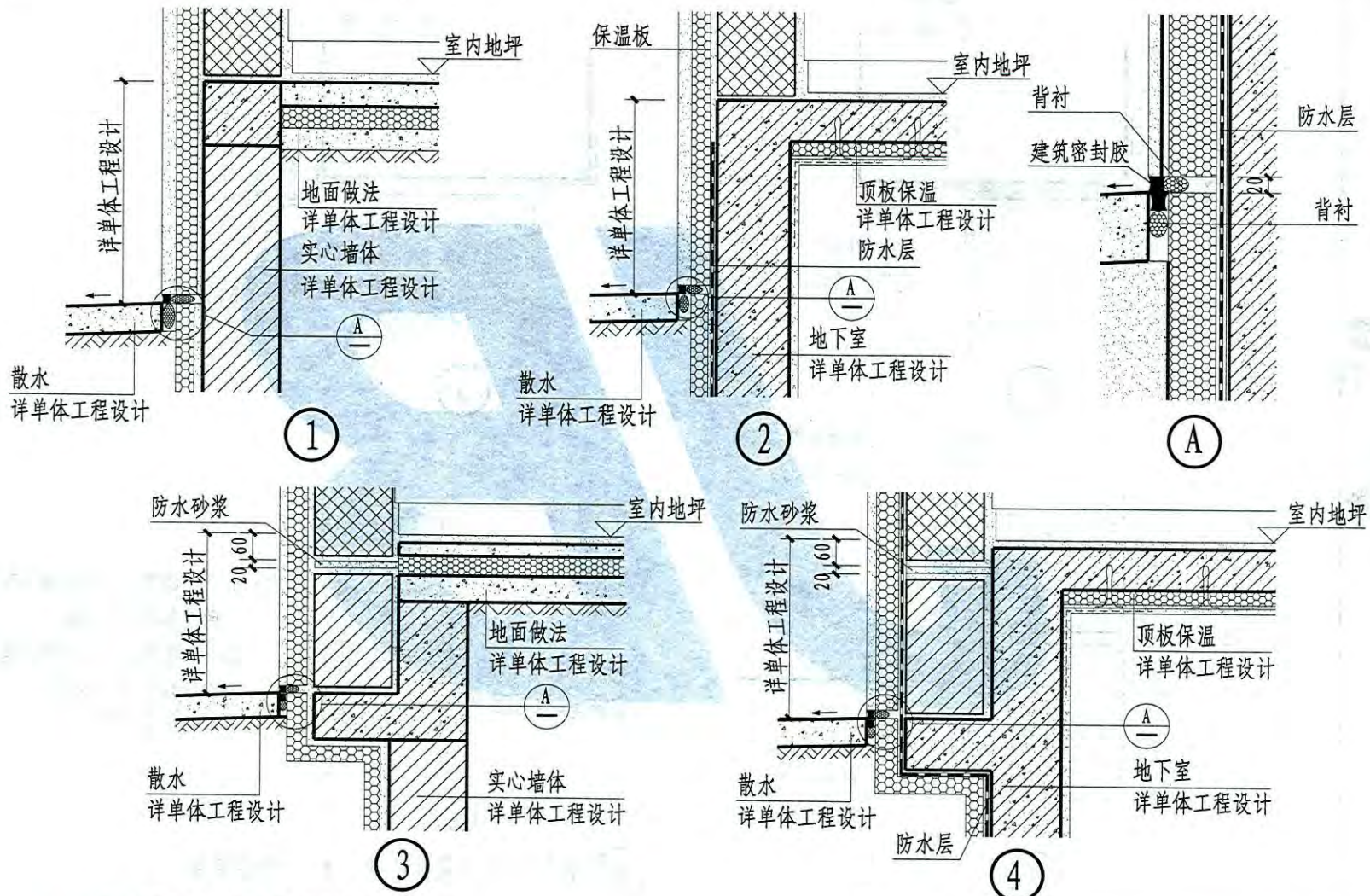
墙身勒脚详图
