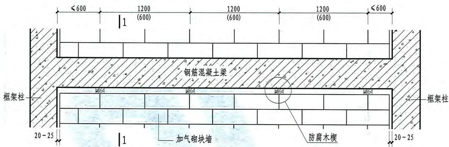
墙顶部连接
