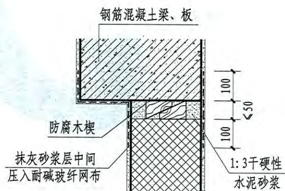
1-1 梁板下墙顶部做法 (平齐)
