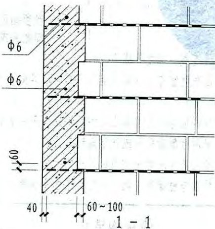
① 砖砌体与加气砌块墙相接
