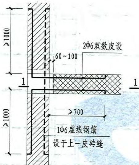
① 砖砌体与加气砌块墙相接
