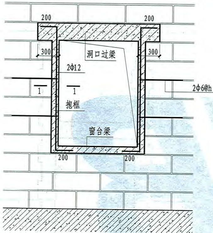
洞口宽度 \leq 2100 窗洞口做法 (一)
