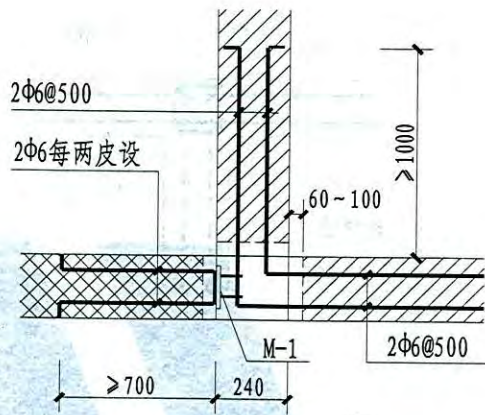
② 构造柱与后砌加气砌块墙相接
