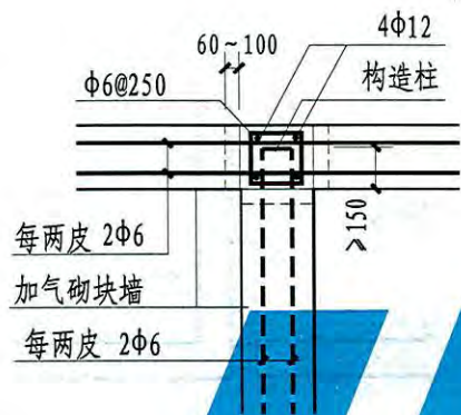
② 构造柱及与墙体拉结图
