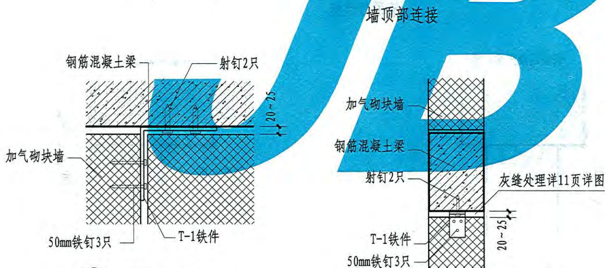
① 梁板下墙顶部做法
