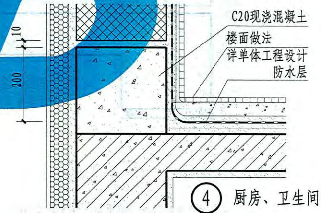
② 厨房、卫生间楼面防水
