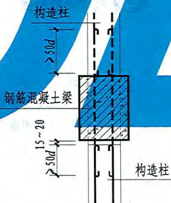
④ 构造柱顶与钢筋混凝土梁 连接处做法
