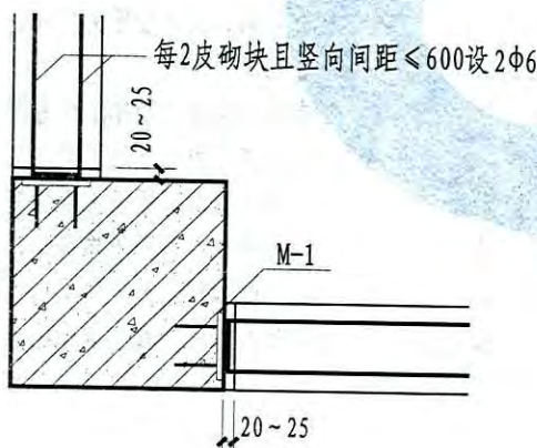
③ 平齐角柱墙
