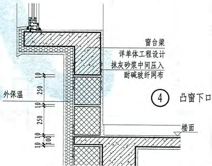
窗上口、窗下口构造详图（一）
